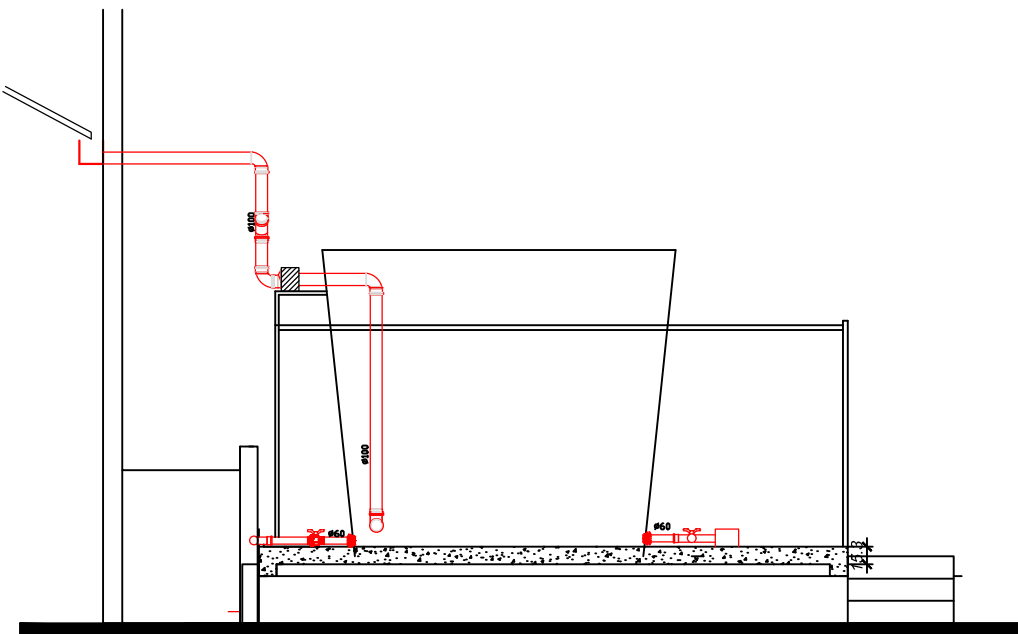
CORTE BB
