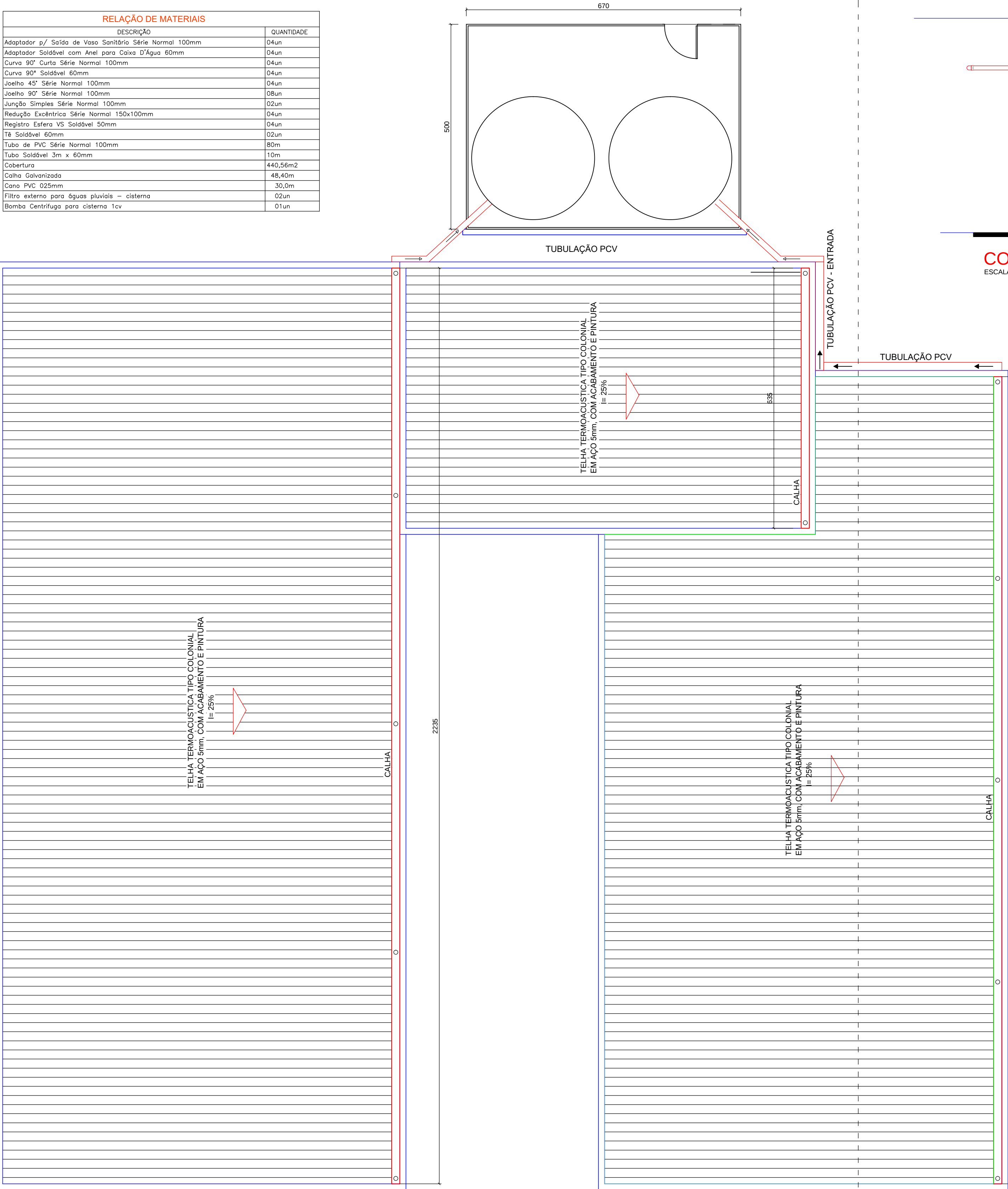
PLANTA BAIXA - CORBERTURA
