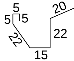
DETALHE CALHA
