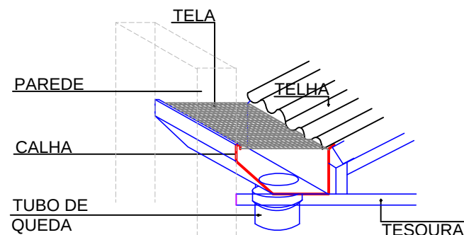
DETALHE CALHA
