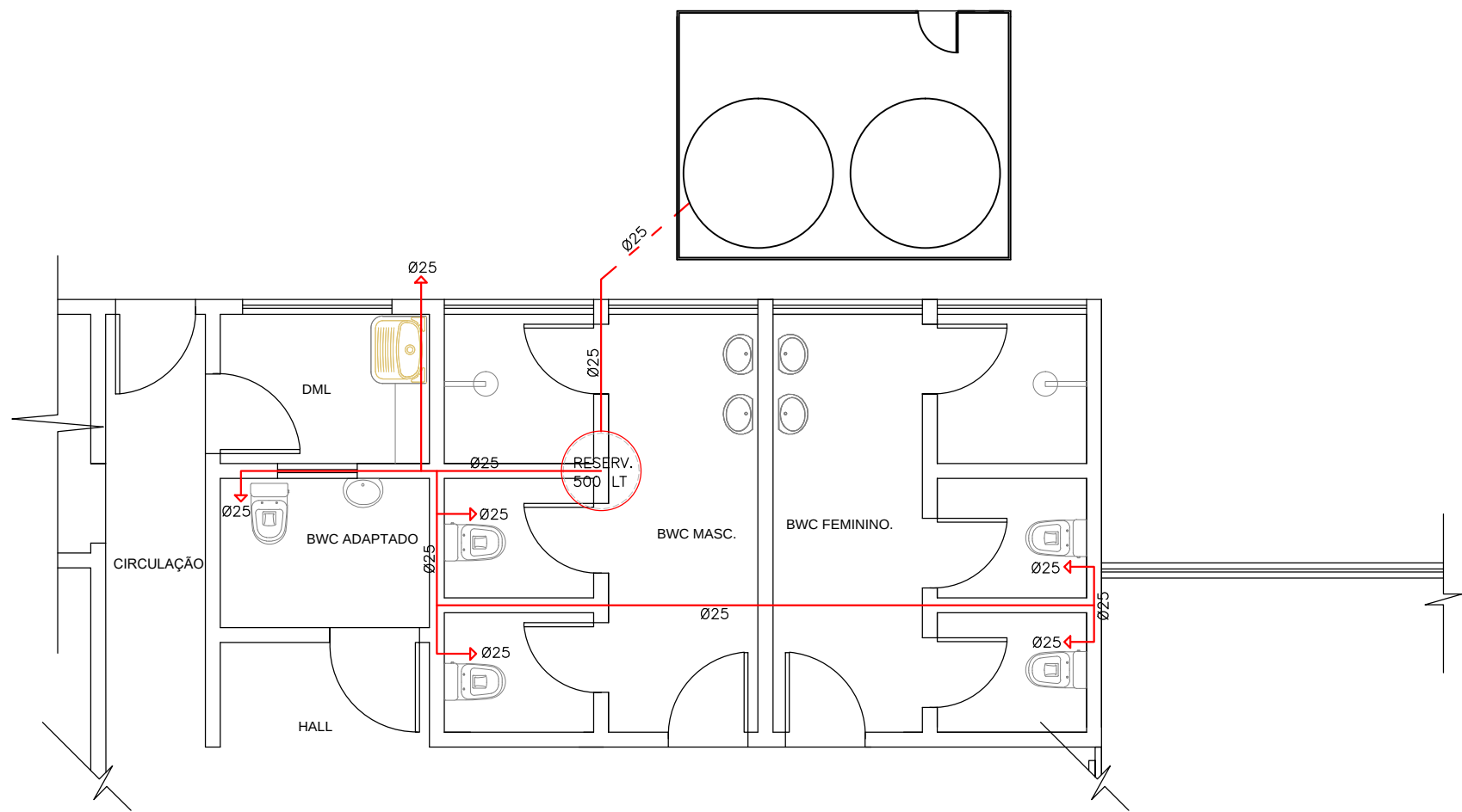
DETALHE - DISTRIBUIÇÃO ÁGUA DA CISTERNA
