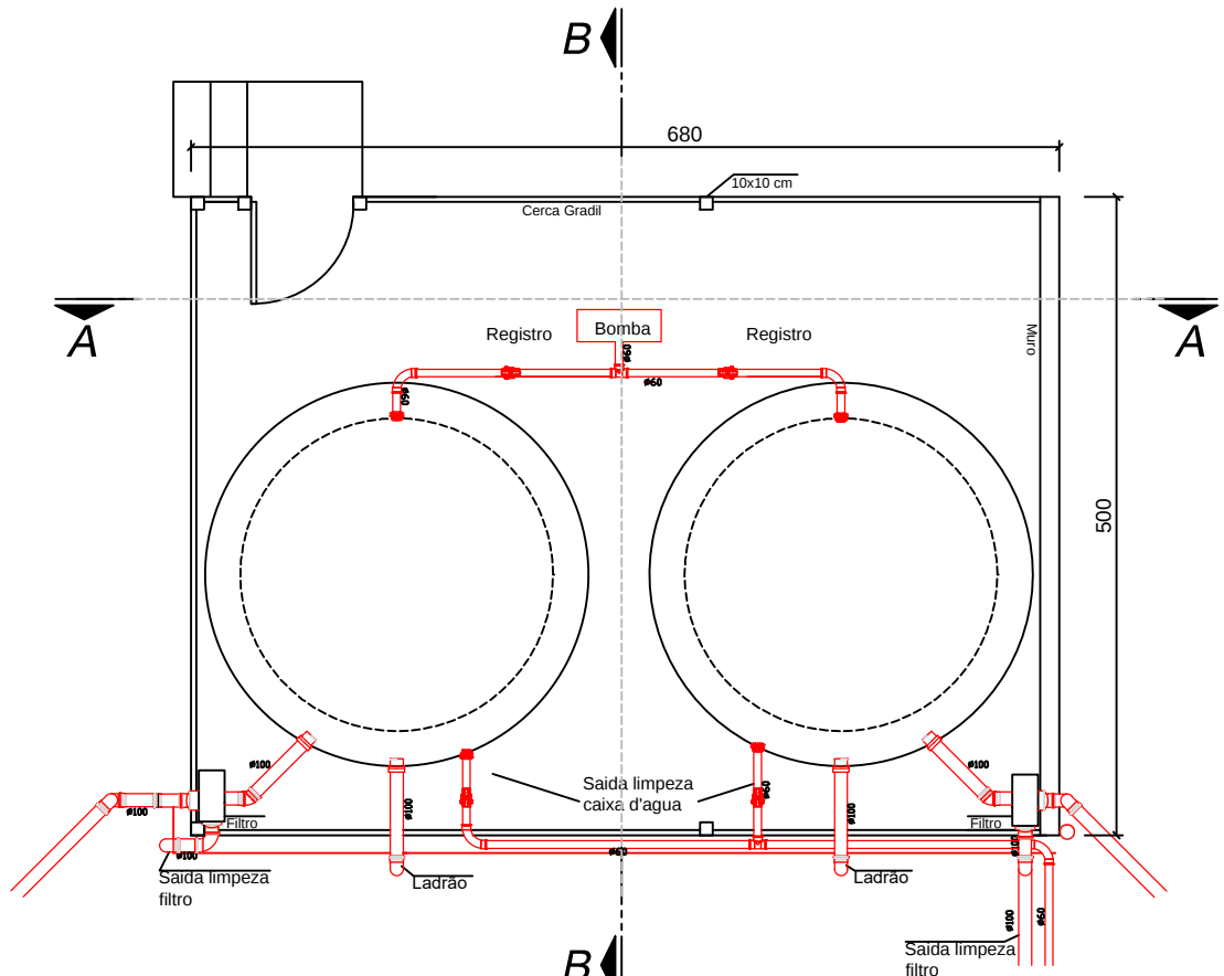
PLANTA BAIXA
